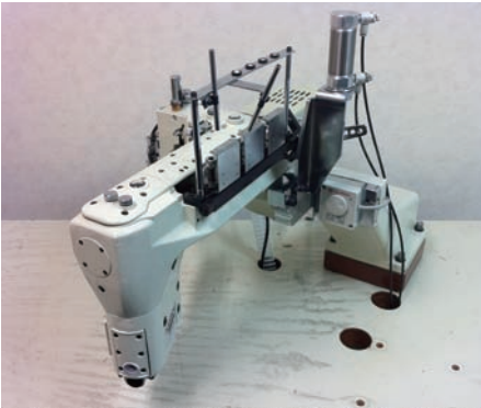
デジタルプーリー (ダイレクトモーター取付時) digital pulley (in case of direct motor attached "Direct motor")
