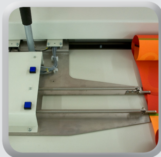
El material se pinza al inicio y al final. Así la posición exacta de la coligación del material está garantizada durante todo el proceso de costura.
